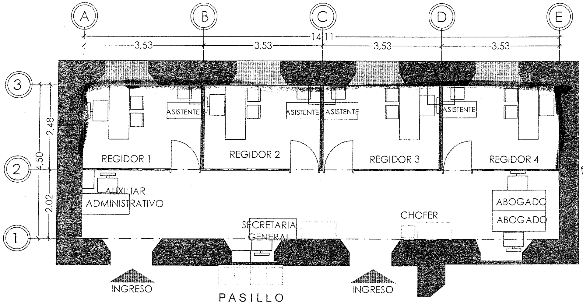
REGIDORES 1 Remodelación H. Ayuntamiento de Colima (Actualmente regidores PRI) Planta Arquitectónica
